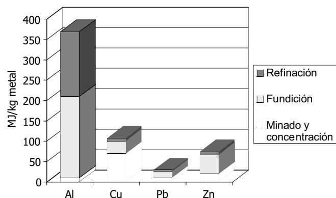
Fig. 2 Consumo específico de energía en la producción de metales.
